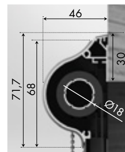
CAJÓN (VISTA LATERAL)
