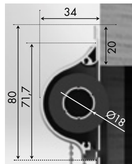
CAJÓN (VISTA LATERAL)
