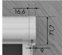
CAJÓN (VISTA FRONTAL)
